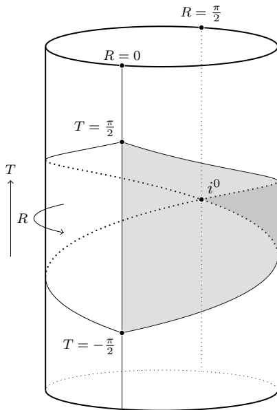
(a) Plongement conforme de Minkowski dans l'espace statique d'Einstein (cylindre).
