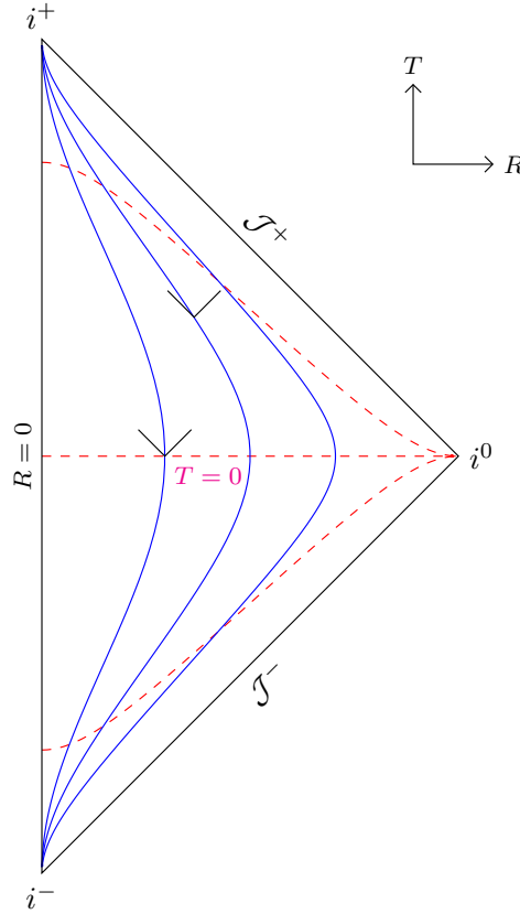
FIGURE 2.12 – Diagramme de Penrose de \mathbb{R}^{1,3} . Ont été indiquées des courbes à r = \text{cste} (bleu) et des courbes à t = \text{cste} (rouge). Ont également été illustrés les cônes de lumière en deux points. Les quantités indiquées sur le bord sont définies ci-dessous, et ne sont pas incluses dans Minkowski.
