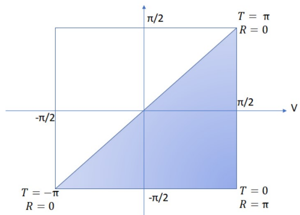
(b) Espace de Minkowski (bleu) dans les coordonnées (U, V) . Note : les coordonnées (T, R) sont ici changés d'un facteur 2.
